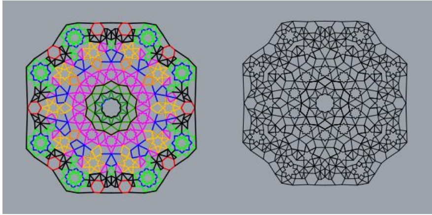
Şekil 13: Sahip Ata camii mukarnasının geometrilerinin belirlendiği plan şeması
