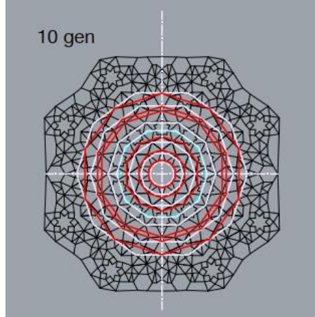
Şekil 14: Sahip Ata camii mukarnasının geometrilerinin katmanları
